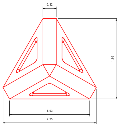
平面図
